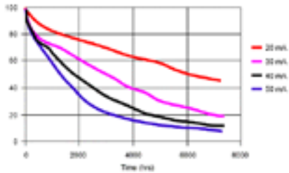
Tablica slabljenja inteziteta svjetla u odnosu na sate rada.
